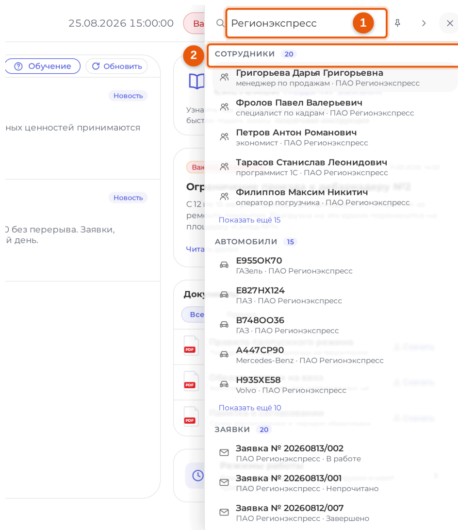
Рисунок 4.4 — Панель поиска
